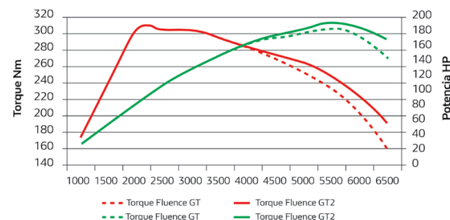
Curva torque y potencia:
